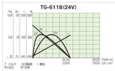
モーター単体負荷特性図
